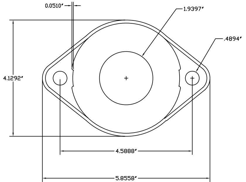
1 1/2" DISCHARGE FLANGE
