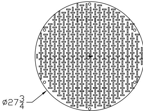
TOP SIDE
